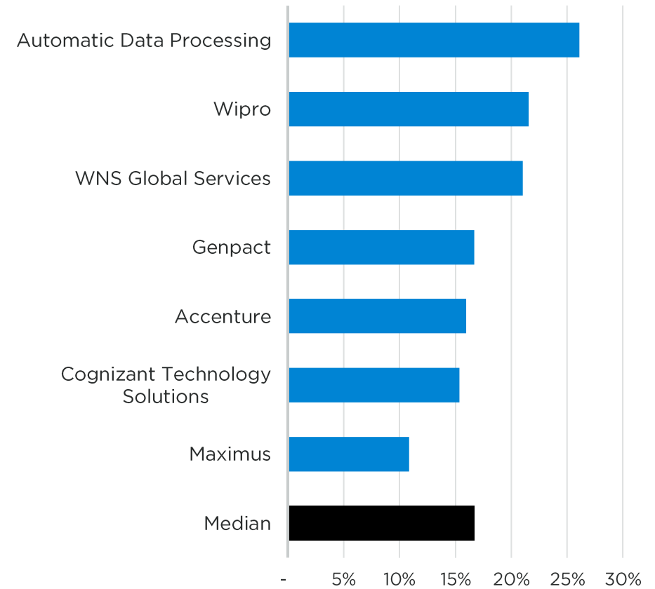
LTM EBITDA %
